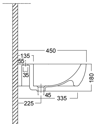
Art. 0450 Lavabo Trinity/ Soho cm.50 Trinity/ Soho wall hung bidet cm.50
